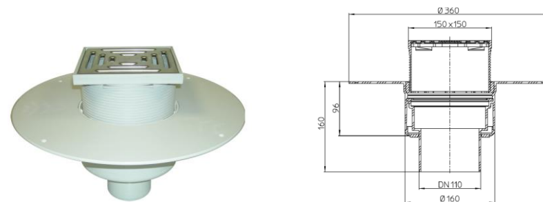
Рис. 2. Кровельная воронка HL62BP/1.
