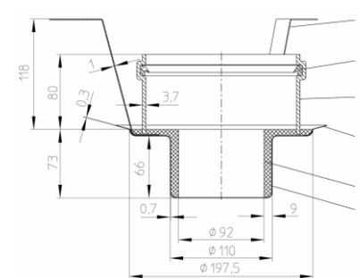
Рис. 4. Противопожарная муфта HL850 для кровельной воронки HL62BP/7.
