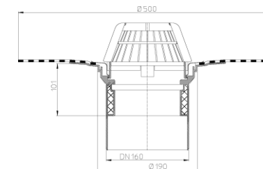
Рис. 1. Кровельная воронка для внутреннего водостока HL62H/5.
