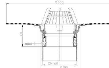
Рис. 1. Кровельная воронка с электрообогревом для внутреннего водостока HL62.1H/5.
