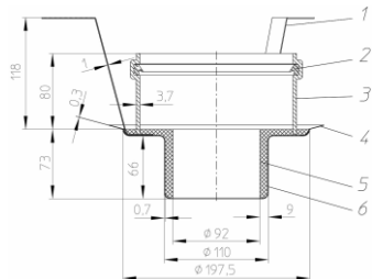
Рис. 5. Противопожарная муфта HL850 для кровельной воронки HL62.1BH/7.
