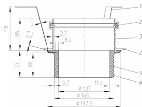
Рис. 6. Противопожарная муфта HL870 для кровельной воронки HL62.1BH/1.
