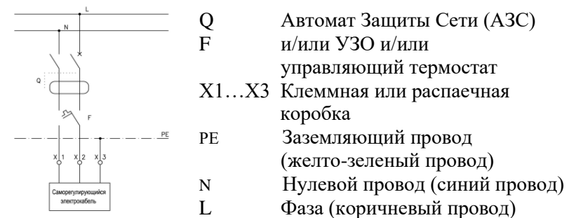
Рис. 4. Схема подключения электрообогрева кровельной воронки HL62.1BH к электрической сети.
