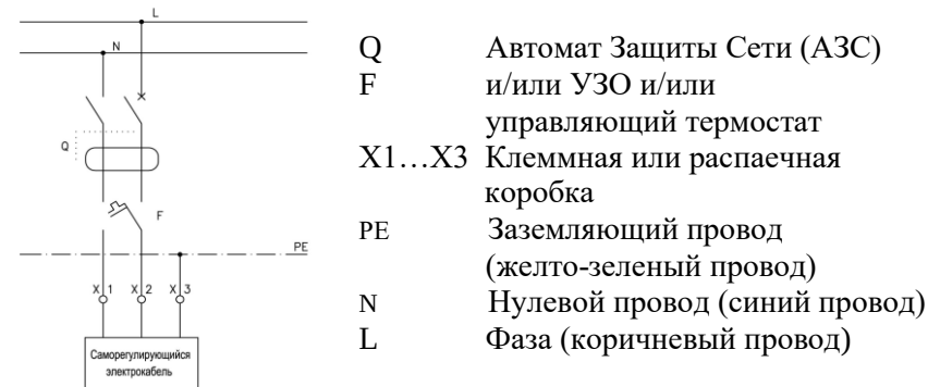
Рис. 4. Схема подключения электрообогрева кровельной воронки HL62.1H к электрической сети.
