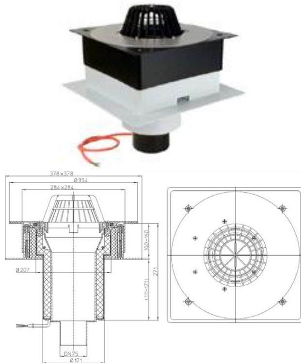
Рис. 1. Кровельная воронка HL63.1P/7.
