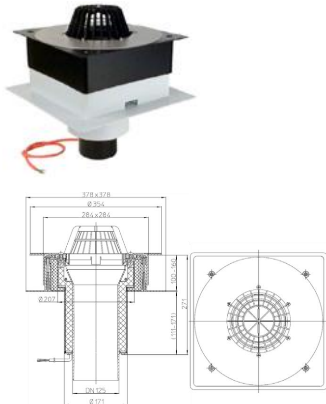
Рис. 3. Кровельная воронка HL63.1P/2.
