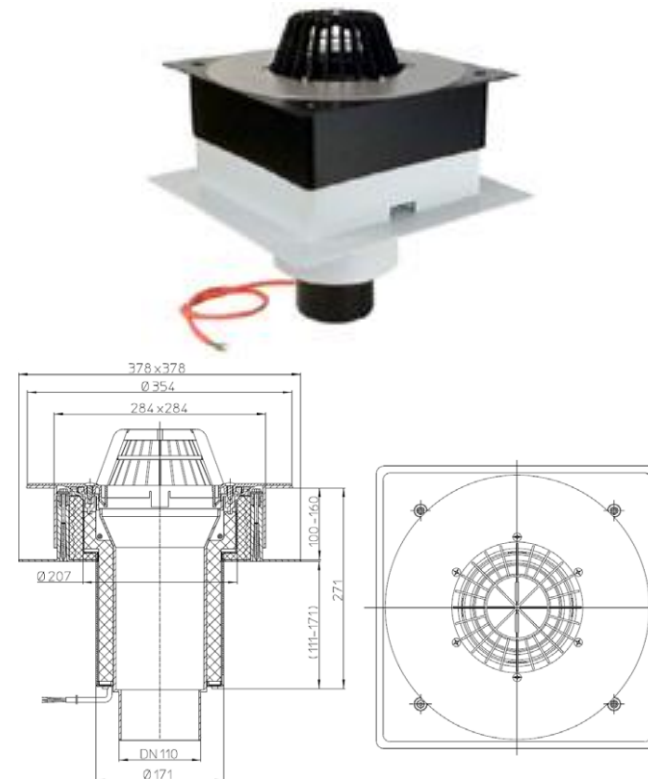
Рис. 2. Кровельная воронка HL63.1P/1.
