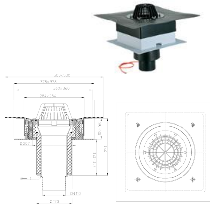
Рис. 2. Кровельная воронка HL63.1H/1.
