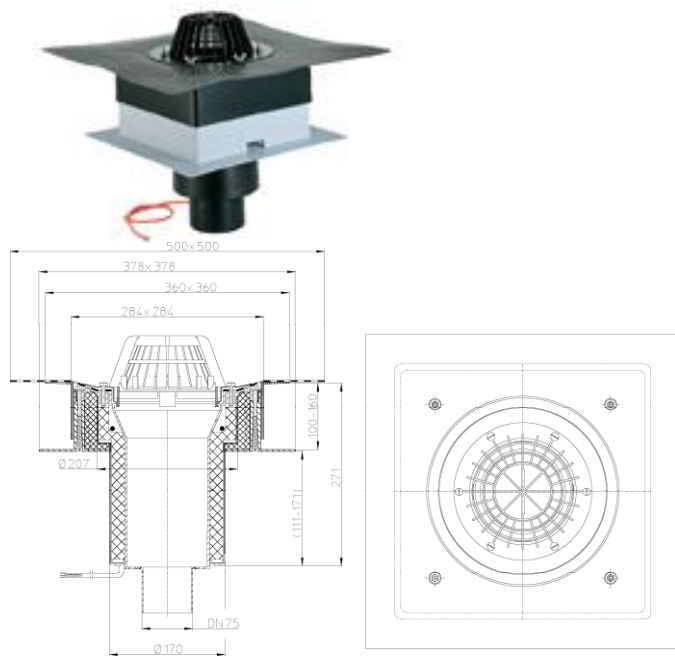
Рис. 1. Кровельная воронка HL63.1H/7.
