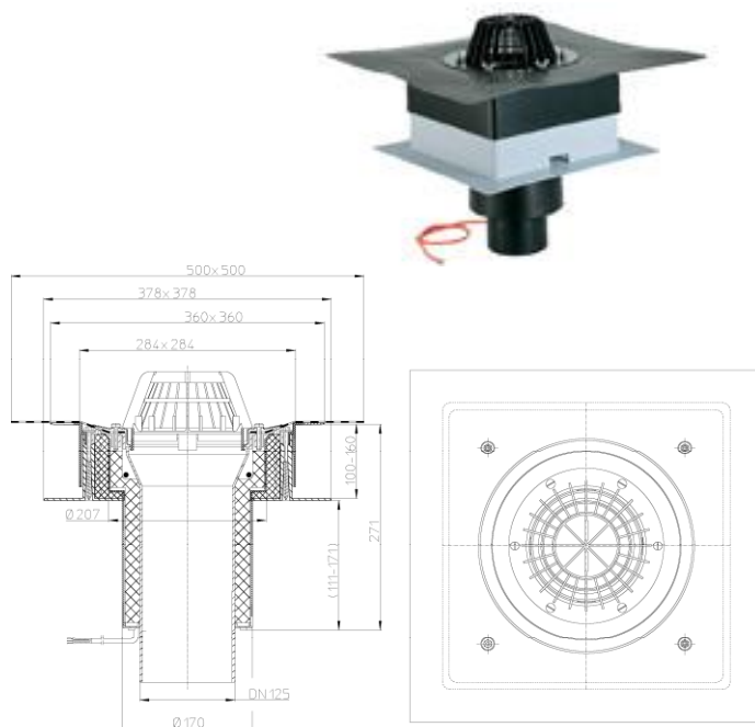
Рис. 3. Кровельная воронка HL63.1H/2.
