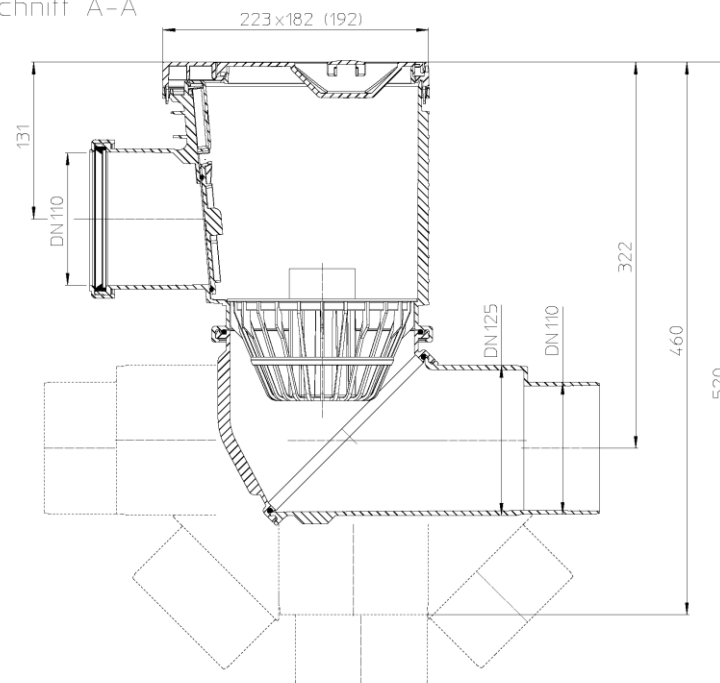
Schnitt A-A
