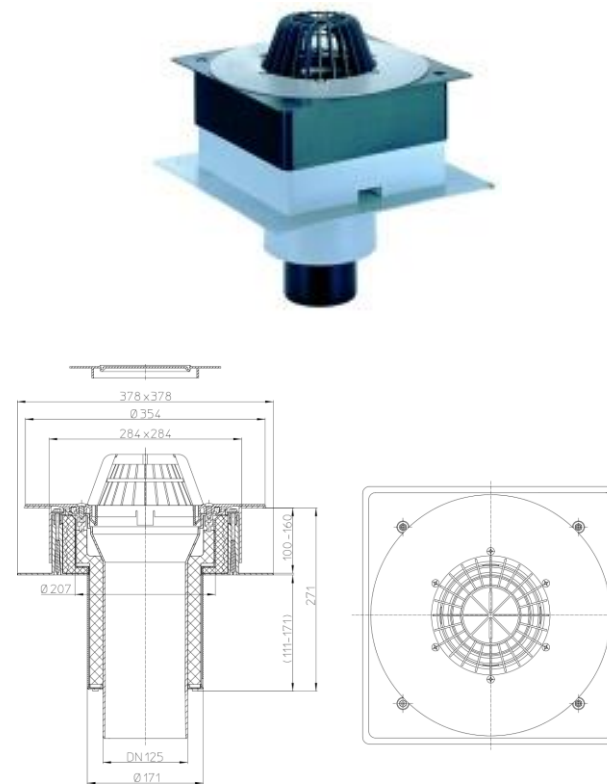
Рис. 3. Кровельная воронка HL63P/2.
