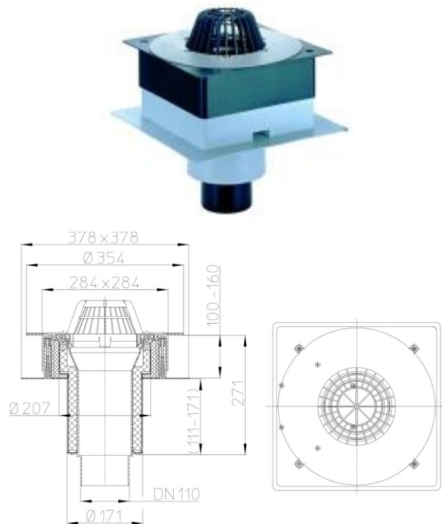
Рис. 2. Кровельная воронка HL63P/1.
