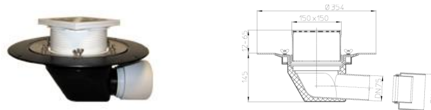
Рис. 1. Кровельная воронка HL64B.
