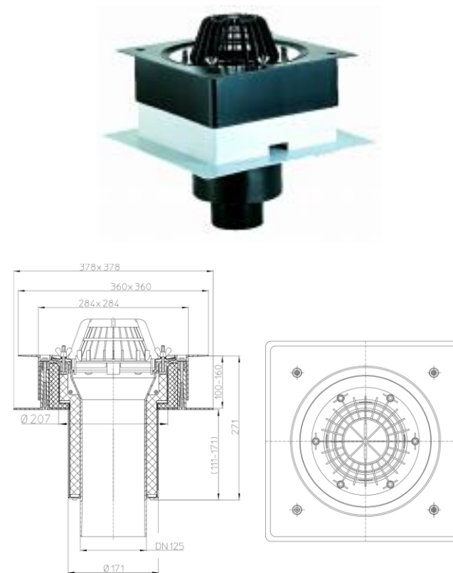
Рис. 3. Кровельная воронка HL63/2.
