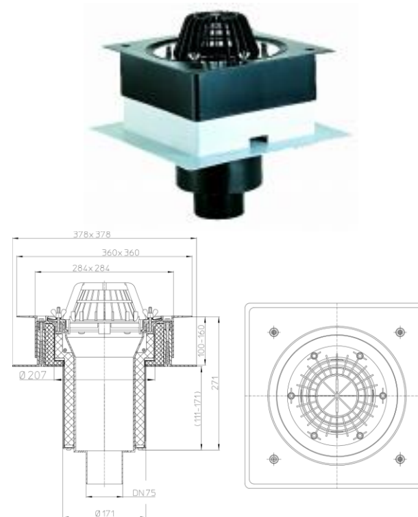
Рис. 1. Кровельная воронка HL63/7.
