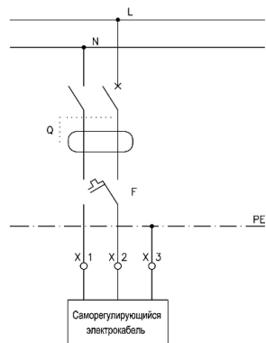
Рис. 2. Схема подключения электрообогрева кровельной воронки HL64.1 к электрической сети.
