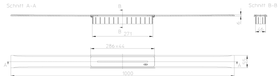
Рис. 1. Декоративная решетка HL053M/100 длиной 1000мм.
