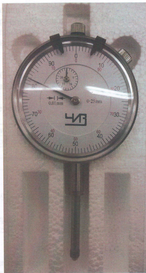
Рисунок 2 – Индикатор часового типа ИЧ 25
