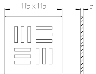
Рис. 7. Декоративная решетка HL3124 (Nil).
