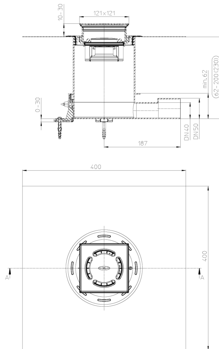
Рис. 1. Трап HL541.
