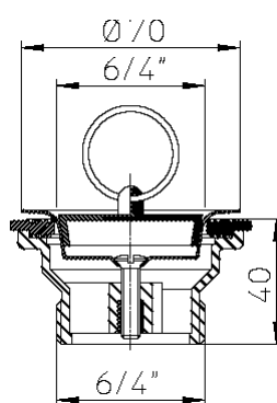
Рис 1. Выпуски для мойки HL15-5/4" и HL15-6/4"
