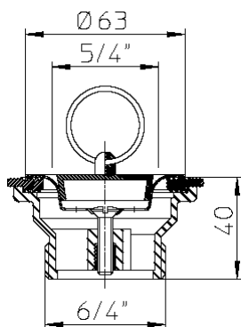
Рис 1. Выпуски для мойки HL15-5/4" и HL15-6/4"
