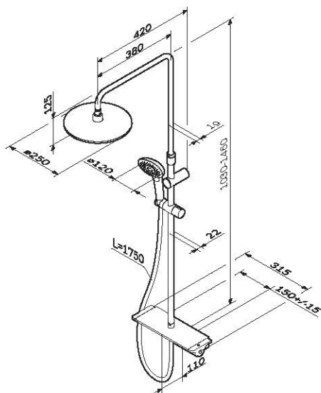
Spirit V2.0 F0770A400
