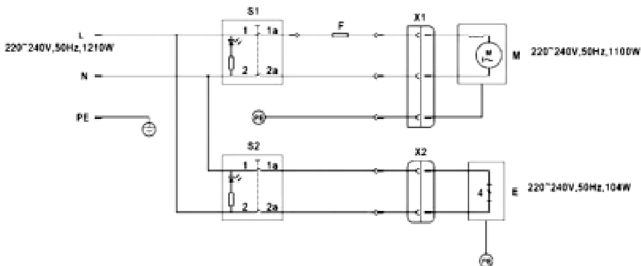
Рис. 3. Электрическая схема.
