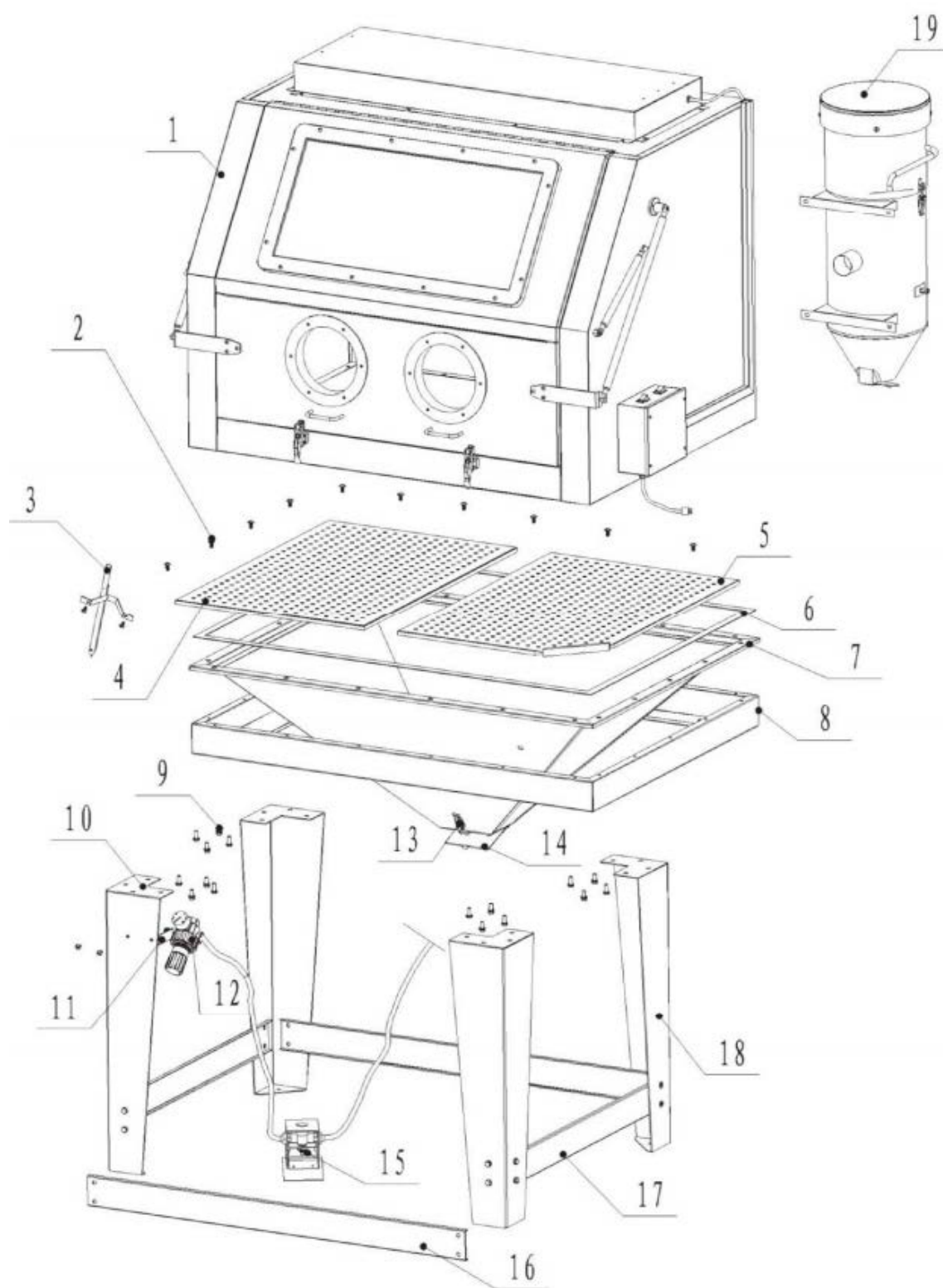
Рис. 2.1. Устройство камеры.
