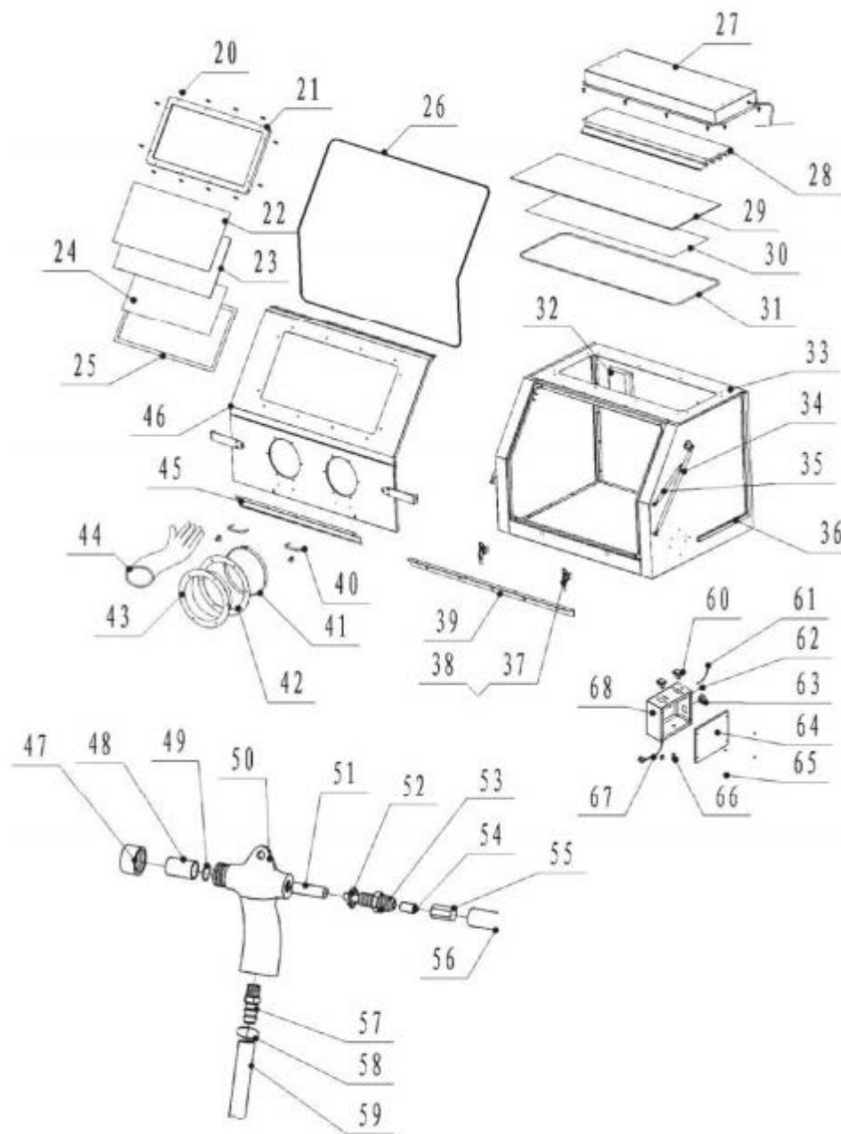
Рис. 2.2. Устройство камеры.
