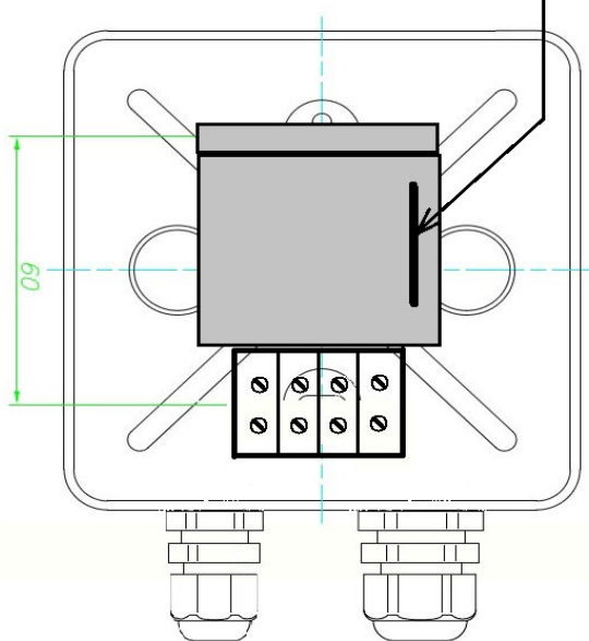
Перемычка
