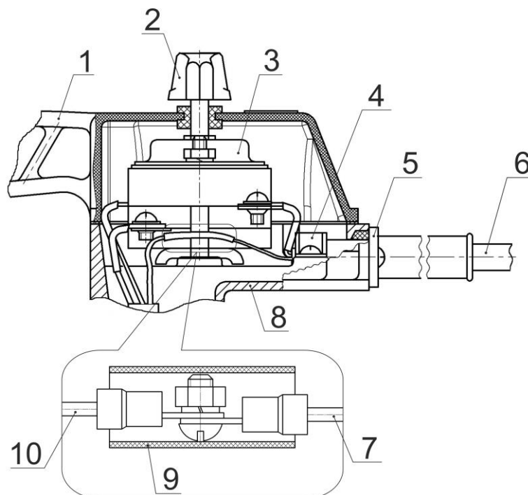
Рисунок 3. Подключение токоподводящего кабеля к электродвигателю вибраторов ИВ-75, ИВ-113, ИВ-116А, ИВ-116А-1.6, ИВ-117А:
