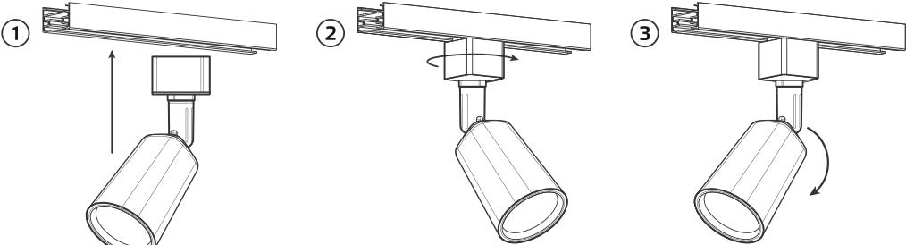
Рис. 1. Порядок монтажа
