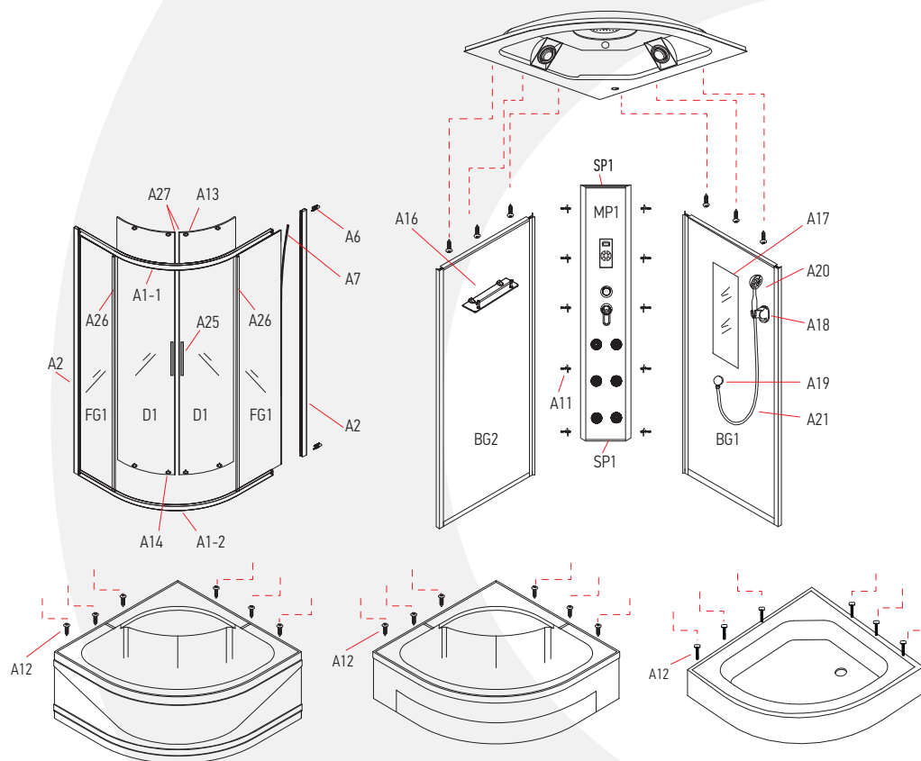
ER35TP/TPF, ER45TP
