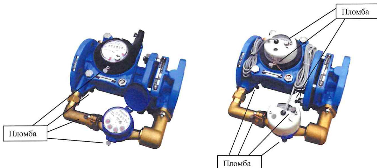
Рисунок 7 - Пломбировка КВСХ-03, КВСХд-03.
