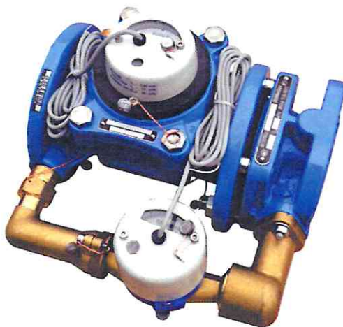
Рисунок 3 - КВСХд-03-80/20
