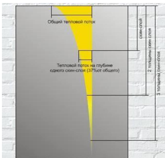
Рис. 1 Изменение интенсивности теплового потока вглубь проводника.
