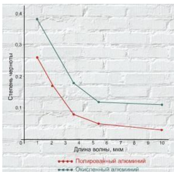
Рис. 2 Зависимость степени черноты от длины волны для полированного и окисленного алюминия.
