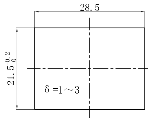
安装面板尺寸 PANEL CUT-OUT
