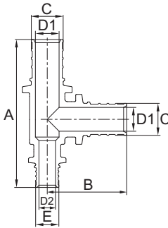
T-Stück mit reduziertem Eingang, axial
