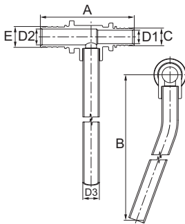
Kühleranschlussrohr T-förmig axial
