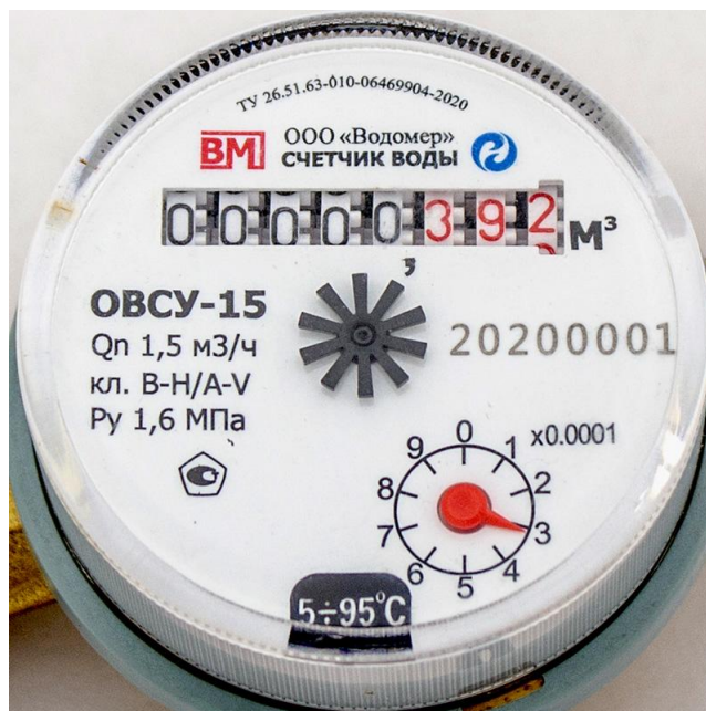
Рисунок 1. Измерительный индикатор счётчика ОВСУ-15
