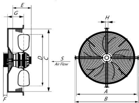
Компактный осевой вентилятор с защитной решеткой YWF S
