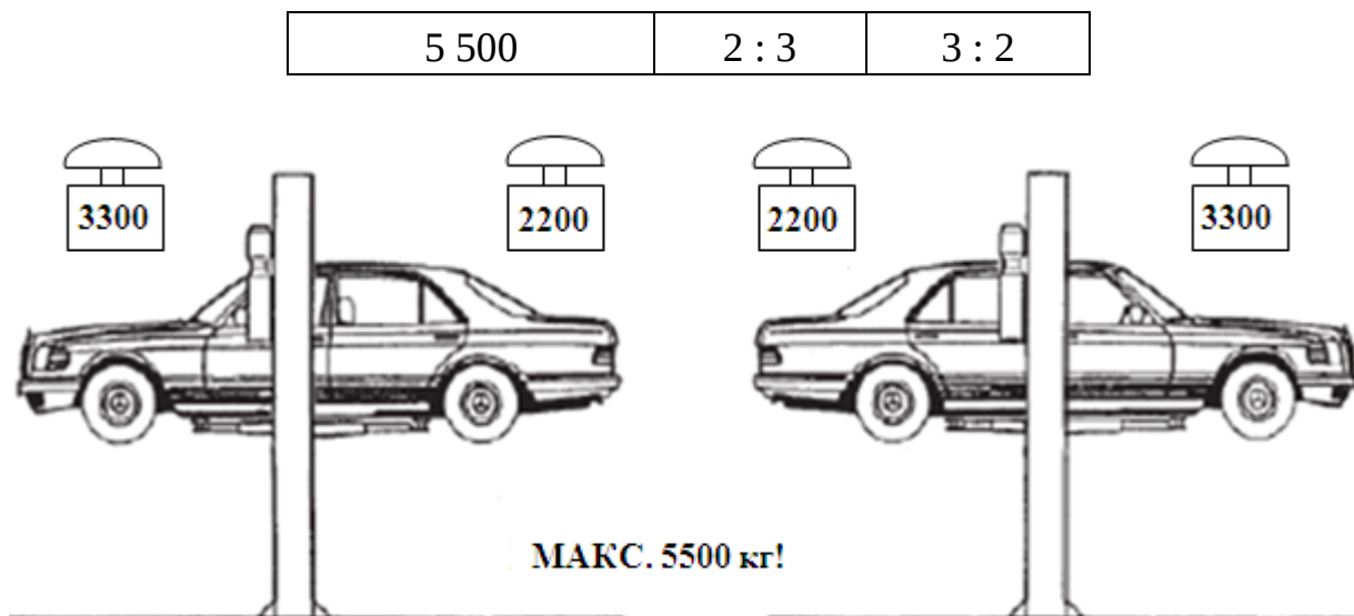
Рис. 20. Распределение веса.
