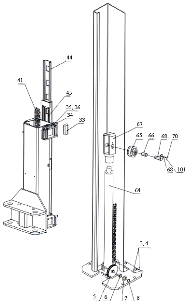
Рис. 11. Узлы и детали подъемника
