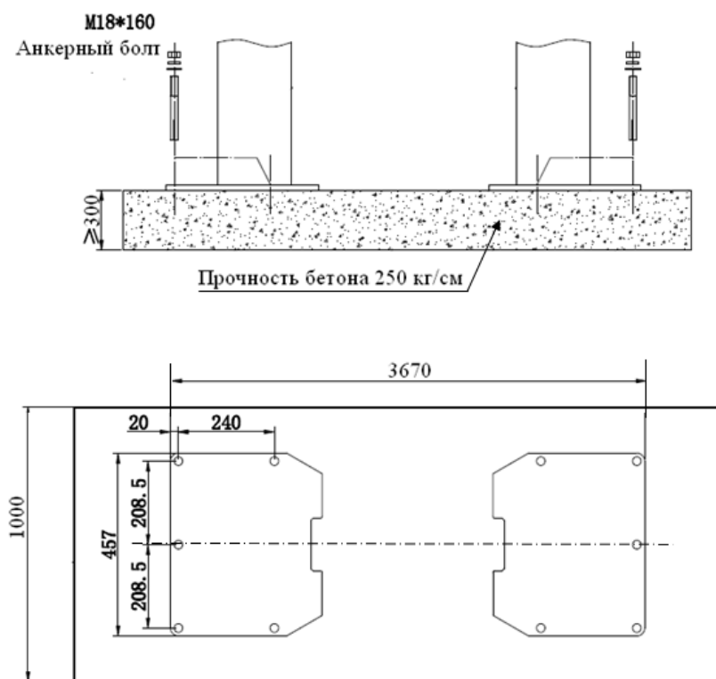
Рис. 2. Фундаментное задание.
