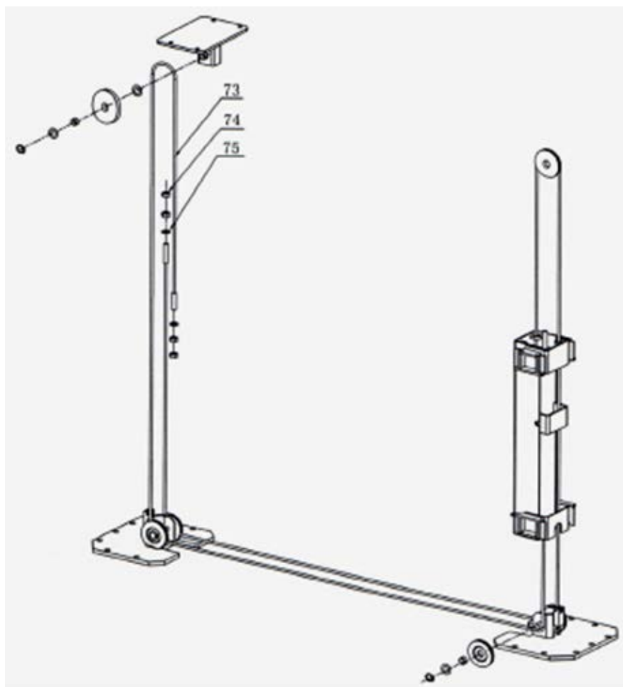
Рис. 13. Узлы и детали подъемника
