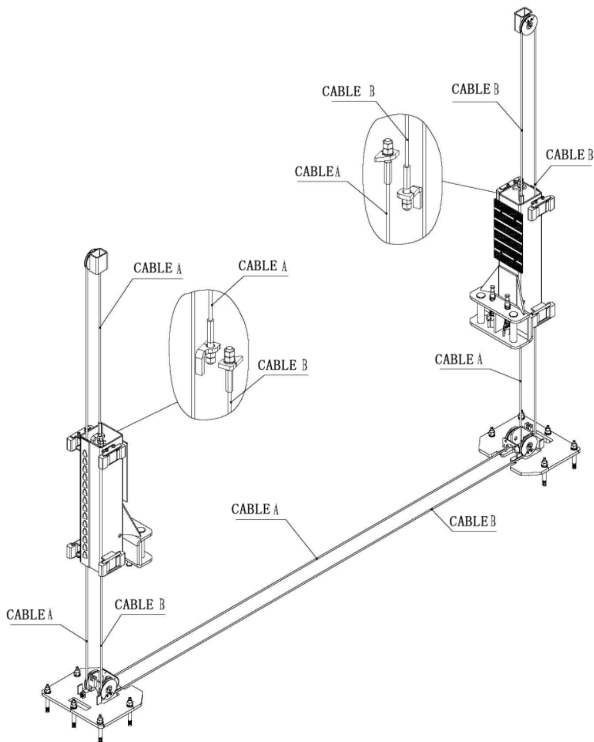
Рис. 14. Система синхронизации кареток
