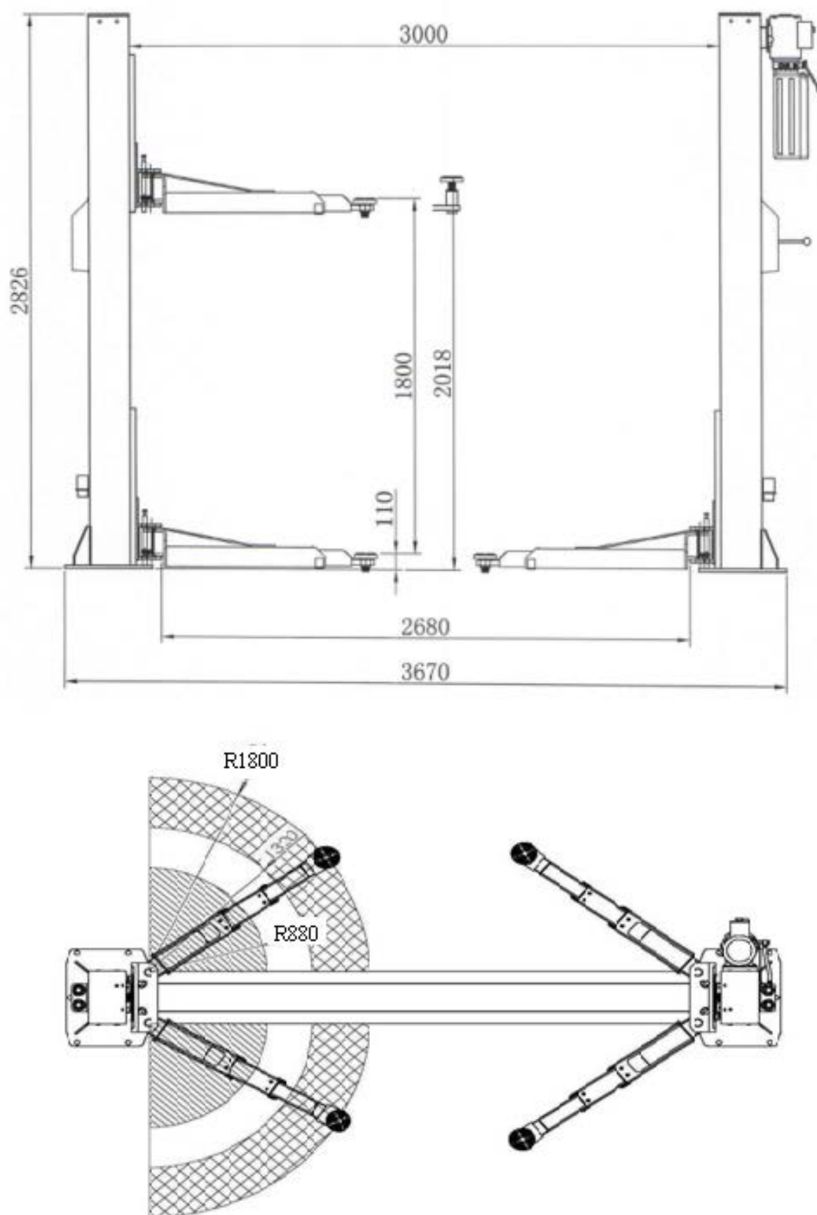
Рис. 3. Габаритные и функциональные размеры.
