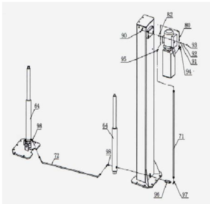
Рис. 12. Узлы и детали подъемника
