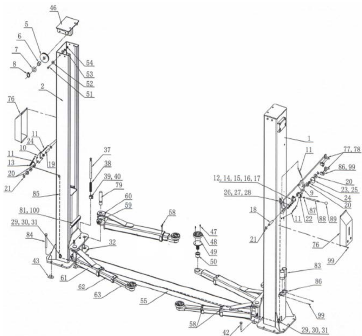
Рис. 10. Узлы и детали подъемника
