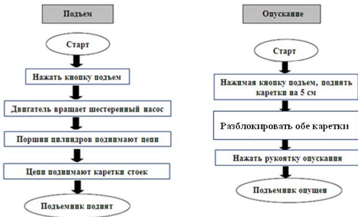
Рис. 6. Блок-схема работы подъемника
