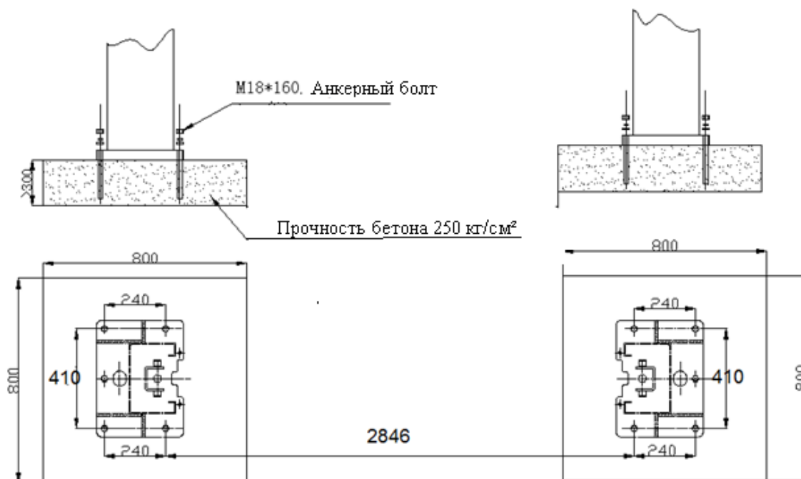
Рис. 1. Фундаментное задание.
