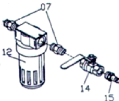
Рис. 5. Сборка влагоотделителя.
