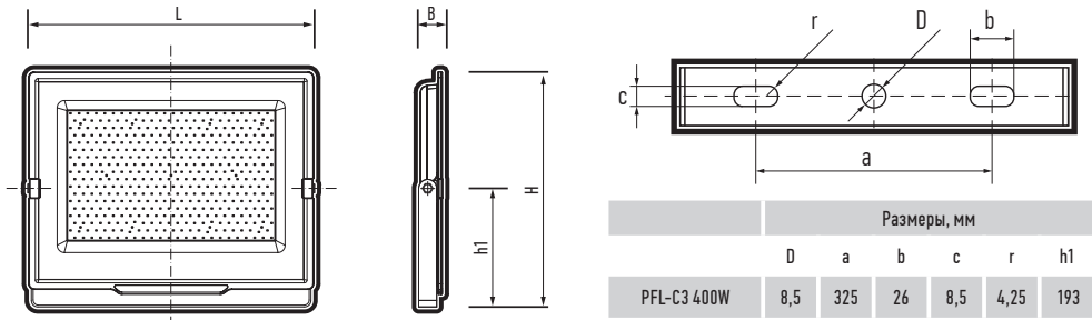
Рис. 1 Прожектор PFL-C3
