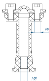
СЕЧЕНИЕ А-А
