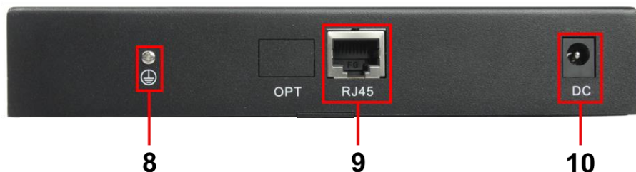
Рис. 3 Передатчик TA-NiKM, разъемы и индикаторы на задней панели
