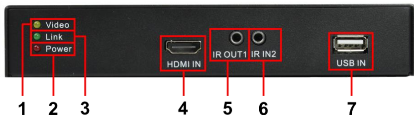
Рис. 2 Передатчик TA-NiKM, разъемы и индикаторы на передней панели
