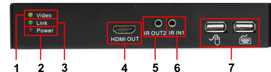
Рис. 4 Приемник RA-HiKM, разъемы и индикаторы на передней панели
