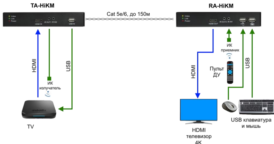
Рис.6 Типовая схема подключения комплекта TA-NiKM+RA-NiKM
