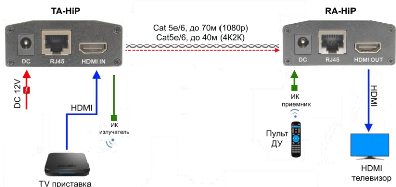
Рис.6 Типовая схема подключения комплекта TA-HiP+RA-HiP
