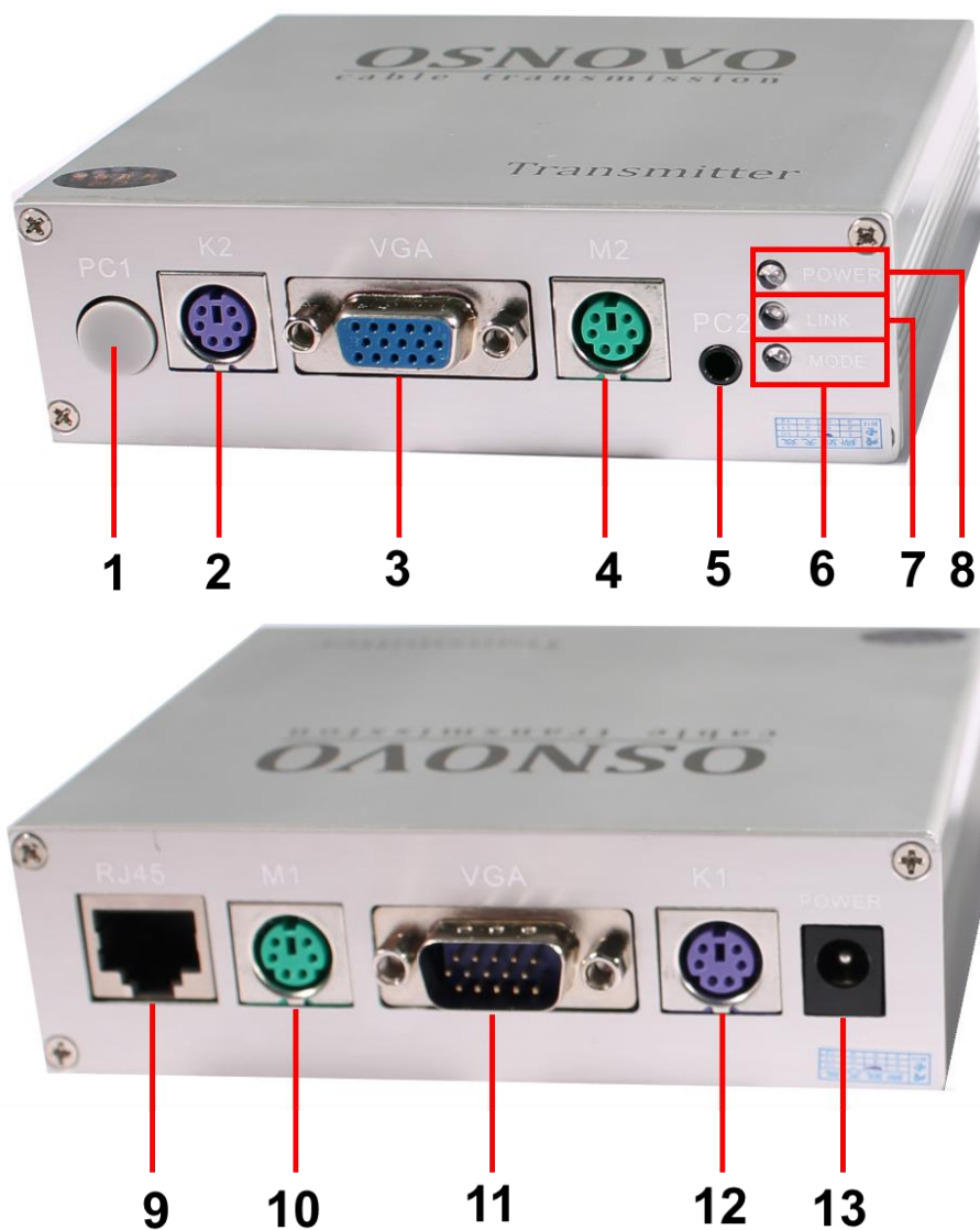
Рис.3 TA-VKM/1, TA-VKM/6, разъемы и индикаторы передней и задней панелей передатчиков
