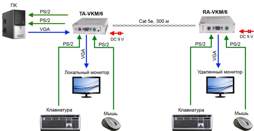
Рис. 10 Схема подключения TA-VKM/6+RA/VKM/6
