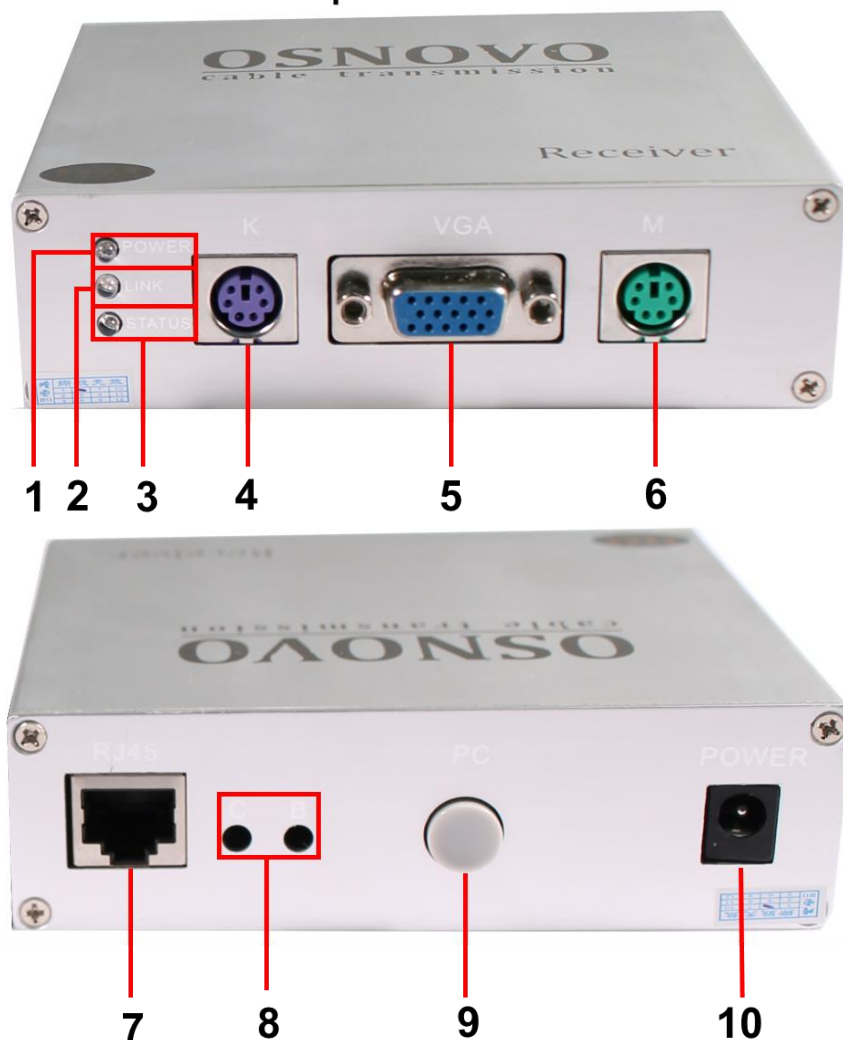
Рис. 4 RA-VKM/1, RA-VKM/6, разъемы и индикаторы передней и задней панелей приемников
