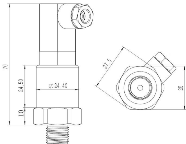
Рисунок 1 – Габаритные размеры
