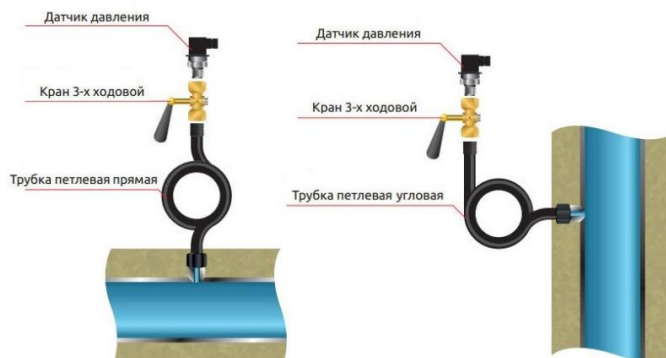
Рисунок 2 – Варианты монтажа на объекте
