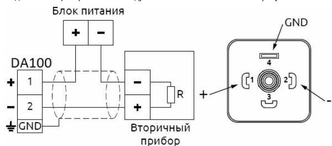
Рисунок 3 – Схема подключения
