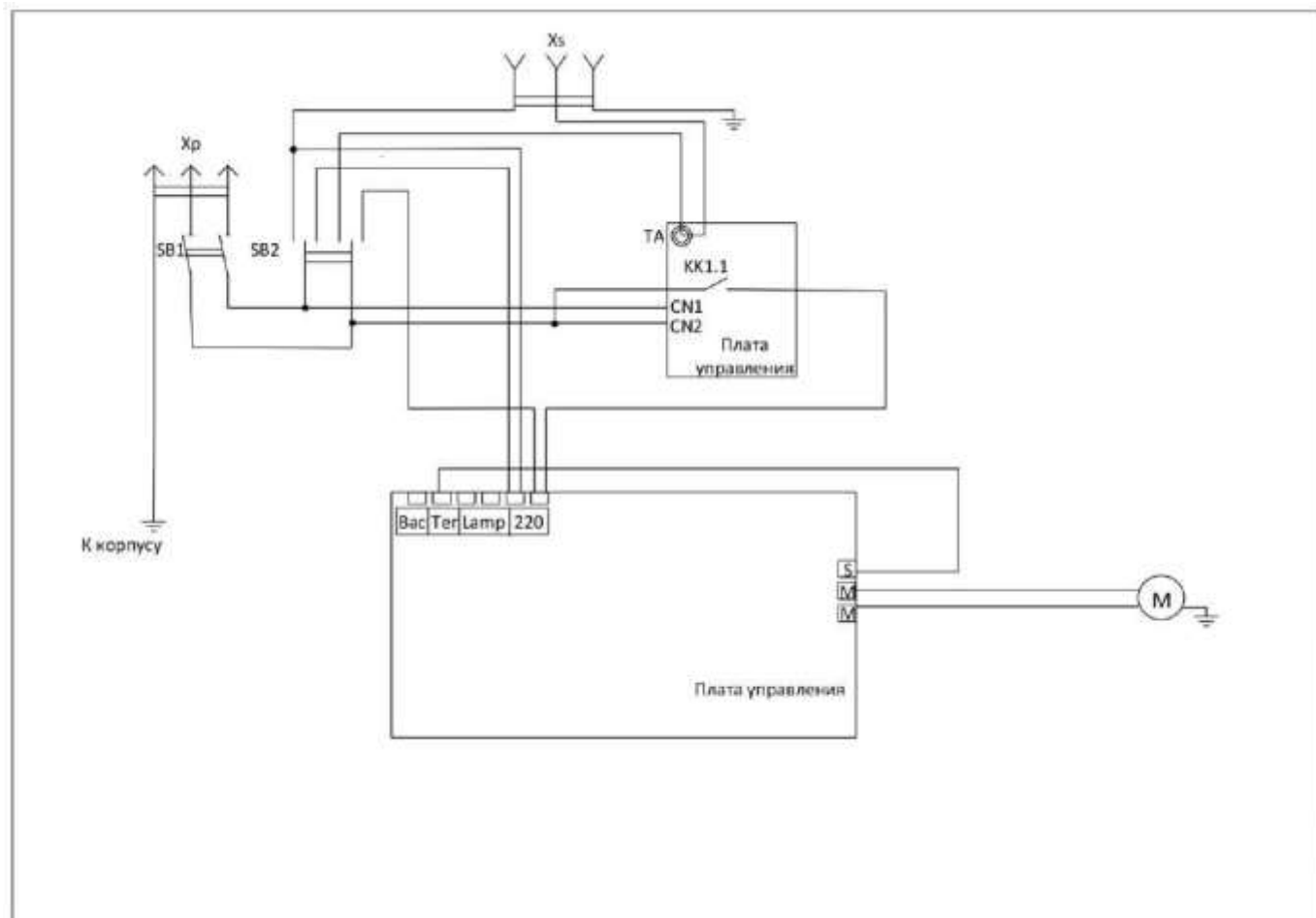
Схема электрическая для моделей ПП-220/15.1, ПП-220/20.6
