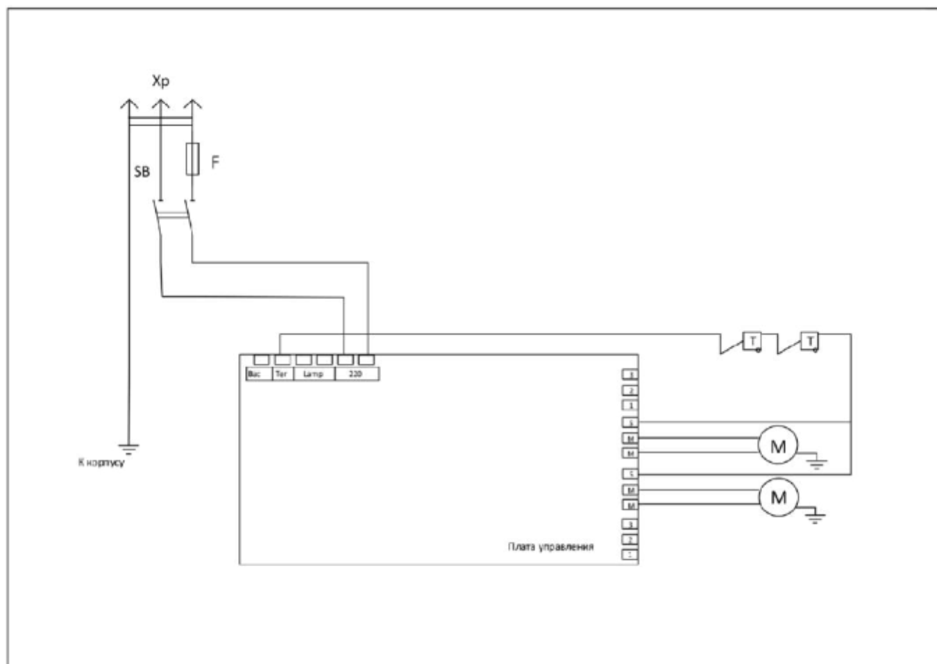
Схема электрическая для модели ПП-220/20.7
