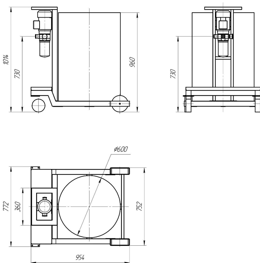
Габаритные размеры.
