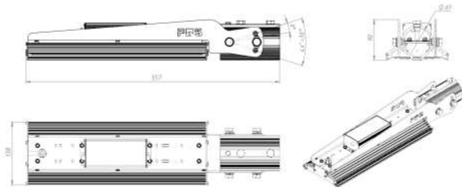
Рис. 1. Габаритные размеры светильника FOS Road R-90
