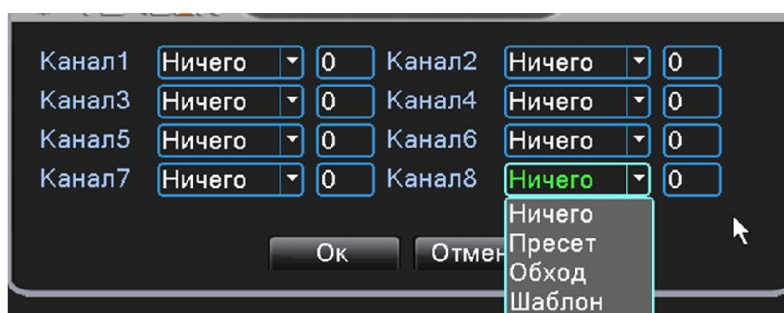
Рис. 4.2.2.3. Тревога. Закрытие камеры. PTZ
