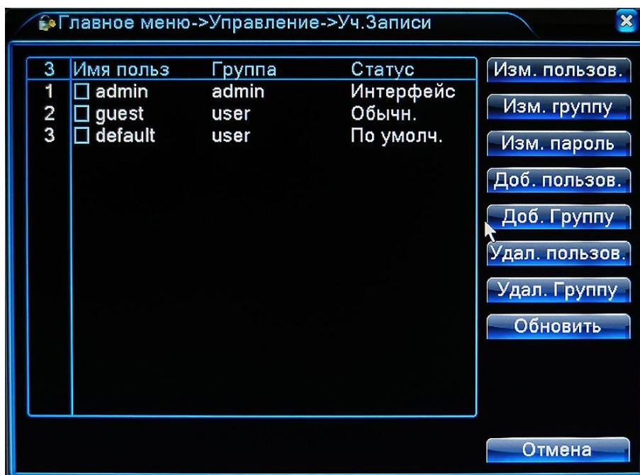
Рис. 4.4.2.1. Управление. Учетные записи
