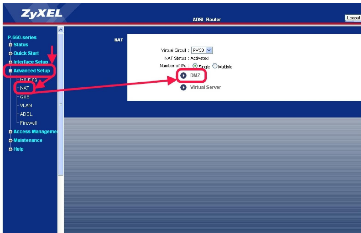
Рис. 6.3. Внесение IP-адреса в DMZ-зону. Стр. 1
