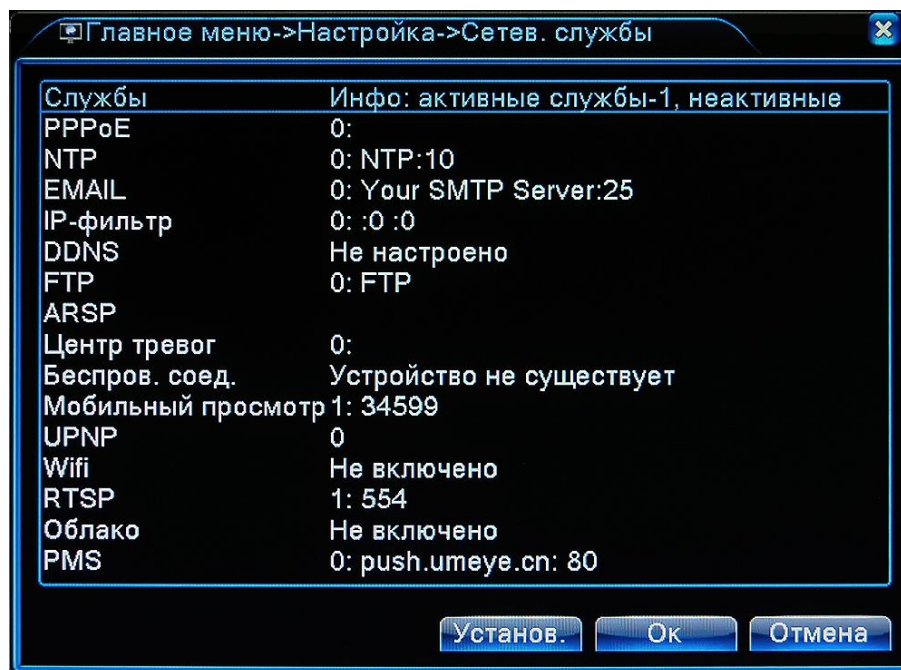
Рис. 4.3.4.1. Настройка. Сетевые службы
