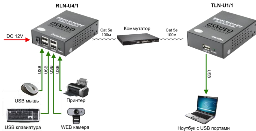
Рис.6 Схема подключения комплекта TLN-U1/1+RLN-U4/1 через сеть на основе коммутатора
