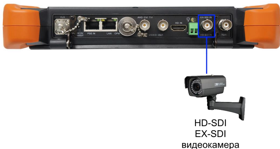
Рис. 13 Подключение EX SDI / HD SDI видеокамеры к тестеру
