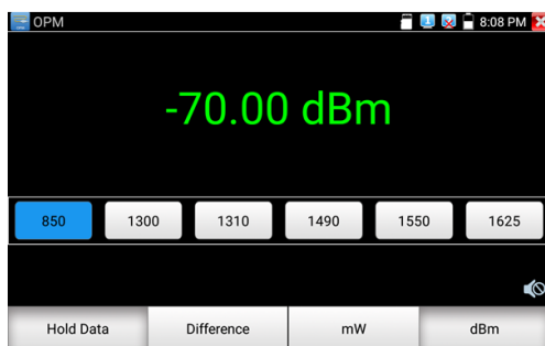
Рис. 131 Использование функции удержания последнего измерения и измерения относительной мощности
