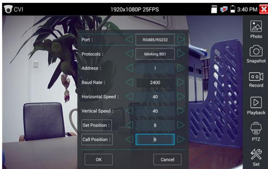
Рис.92 Управление PTZ CVI видеокамерой по интерфейсу RS232/485
