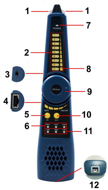
Рис. 114 Мультифункциональный щуп, разъемы и индикаторы
