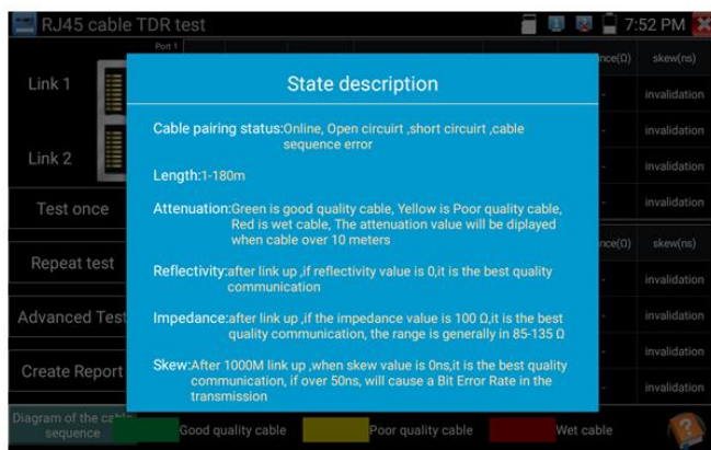
Рис. 118 Справочная информация подключения кабеля к тестеру для TDR теста
