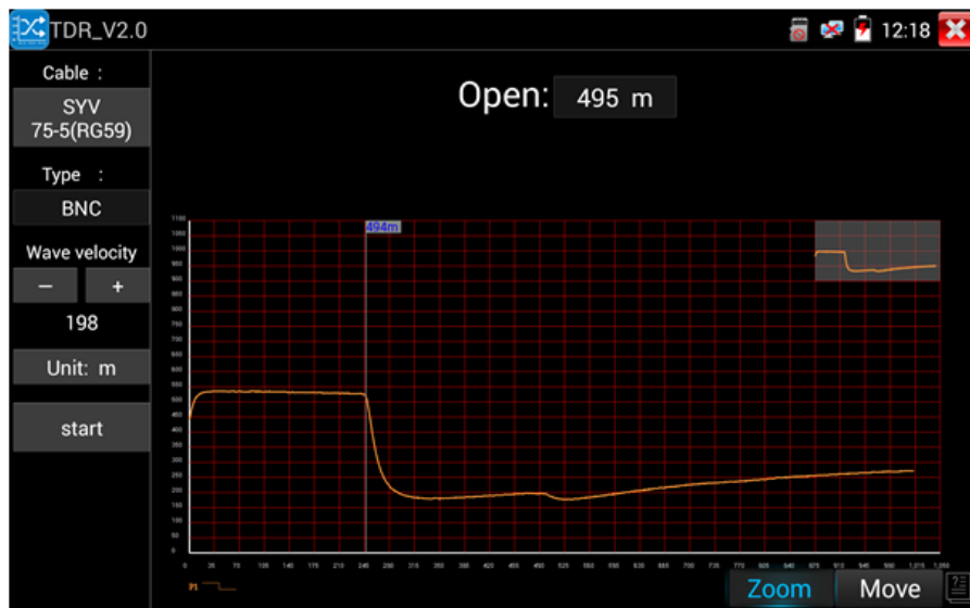
Рис. 120 Рефлектометр (TDR) для коаксиального кабеля, интерфейс
