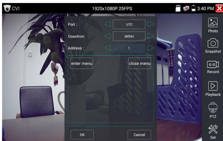
Рис. 93 Настройки для доступа к OSD меню видеокамеры по коаксиальному кабелю
