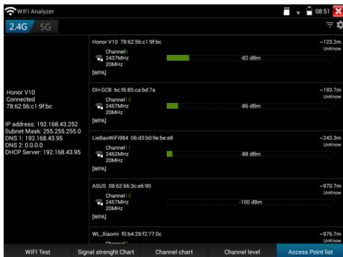
Рис. 159 Интерфейс приложения – анализатора Wi-Fi сетей
