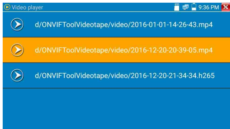
Рис. 48 Меню видеоплеера
