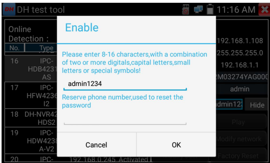
Рис. 148 Установка пароля
