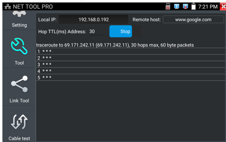
Рис. 110 Интерфейс инструмента «Трассировка маршрута» (Trace Route)
