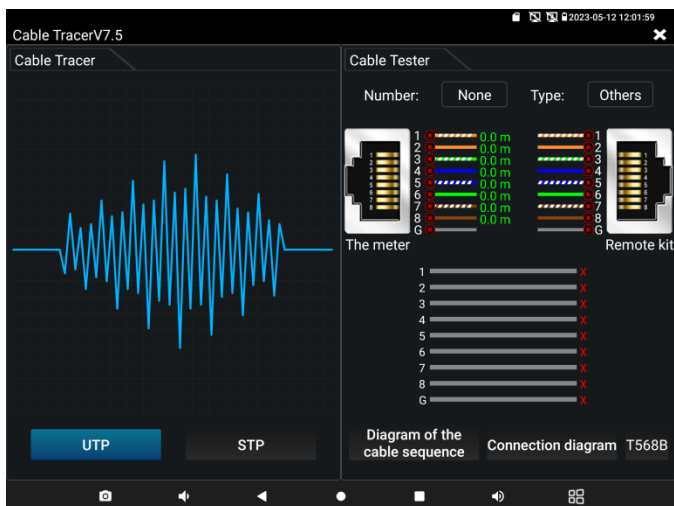
Рис. 115 Интерфейс приложения Cable Tracer
