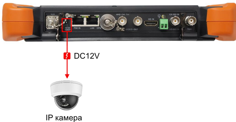
Рис. 9 Подключение питания к IP-видеокамере без PoE
