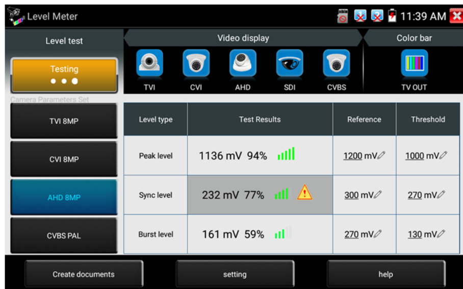
Рис. 84 Интерфейс приложения Level Meter
