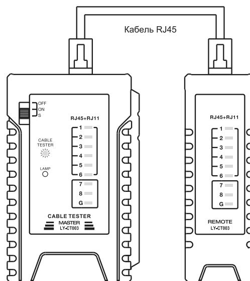
5BITES LY-CT003 Тестер
