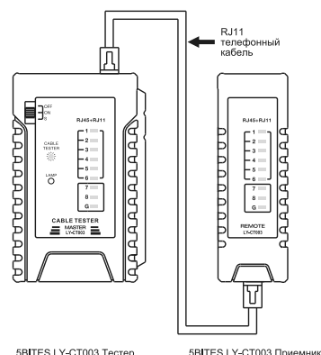
5BITES LY-CT003 Тестер
