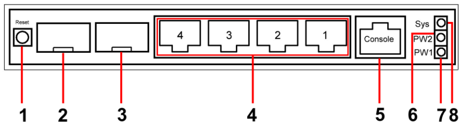
Рис.3 Уличный коммутатор SW-80402/WL, разъемы, кнопки и индикаторы
