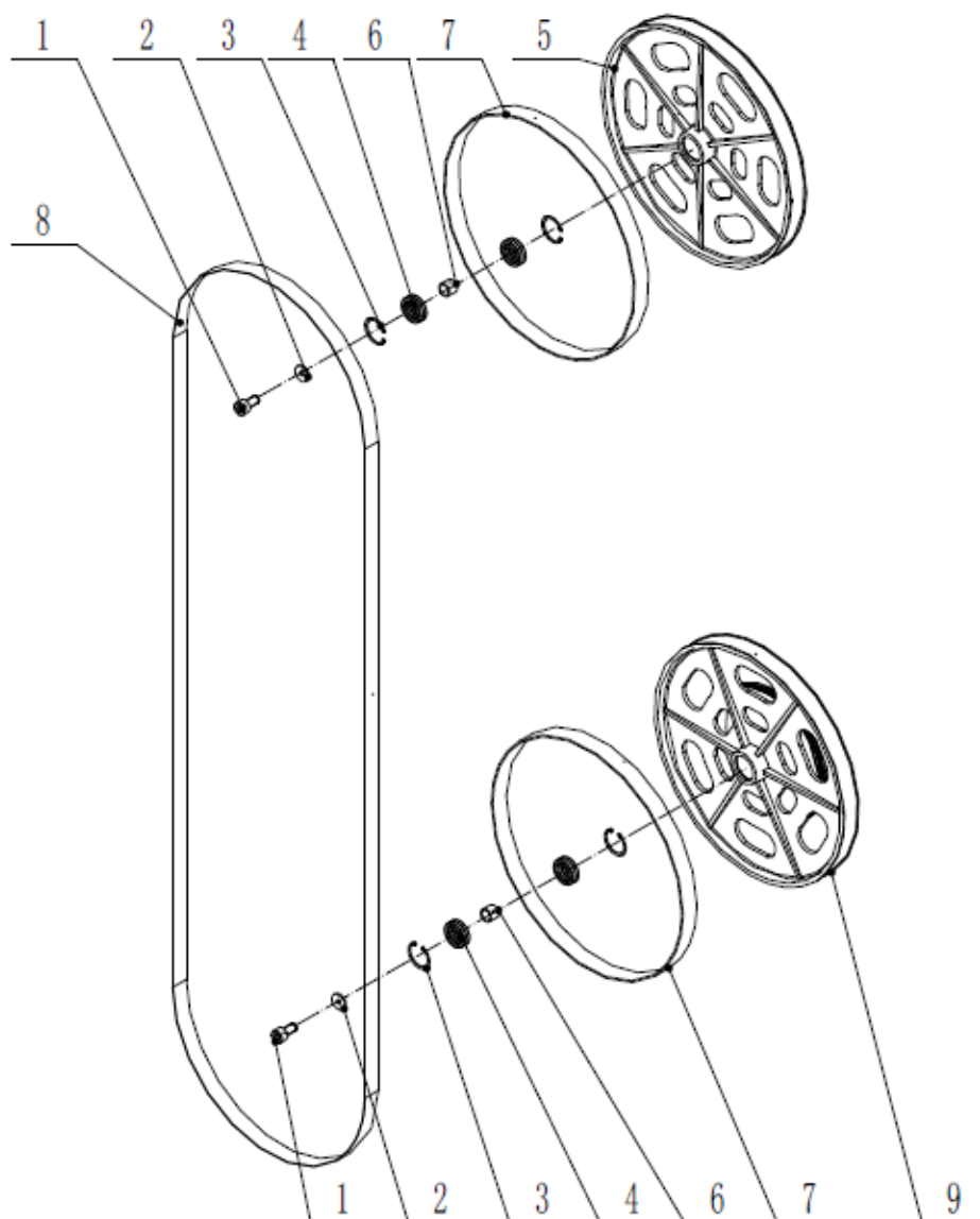
Чертеж В Узел пильного полотна
