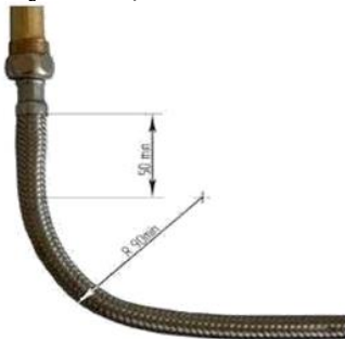
Рис. 4 Требования к монтажу гибких шлангов
