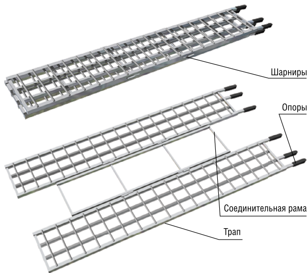
Рисунок 1 – Устройство изделия на основе модели 28.55
