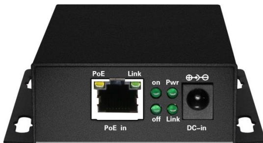
Рис.1 Коммутатор/удлинитель SW-8030/D (вид спереди)
