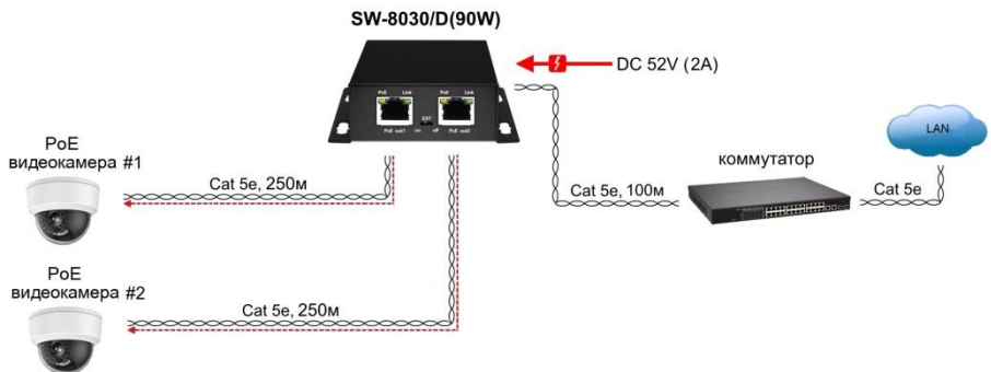
Рис.5 Схема подключения коммутатора/удлинителя SW-8030/D(90W) в режиме увеличения расстояния передачи данных и PoE (до 250м) и питанием от внешнего БП
